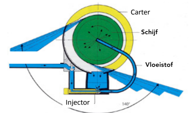
Figuur 19: Roterende schijfvernevelaar
