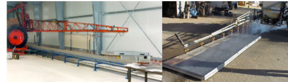
Figuur 24: Testbank om de spuitvloeistofverdeling te controleren
