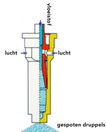
Figuur 15: luchtmengdop
