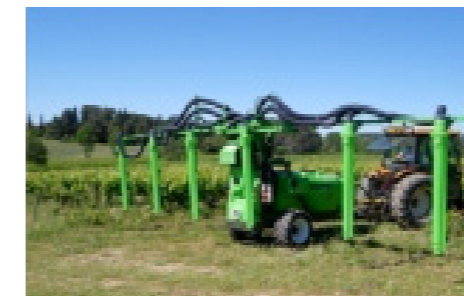
Figuur 17: Meerrijige spuittoestellen, a) met spuitdoppen
